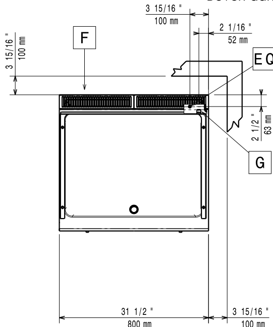
Boven aanzicht
